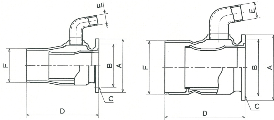
THM型 ミキシング 本体各部寸法表
